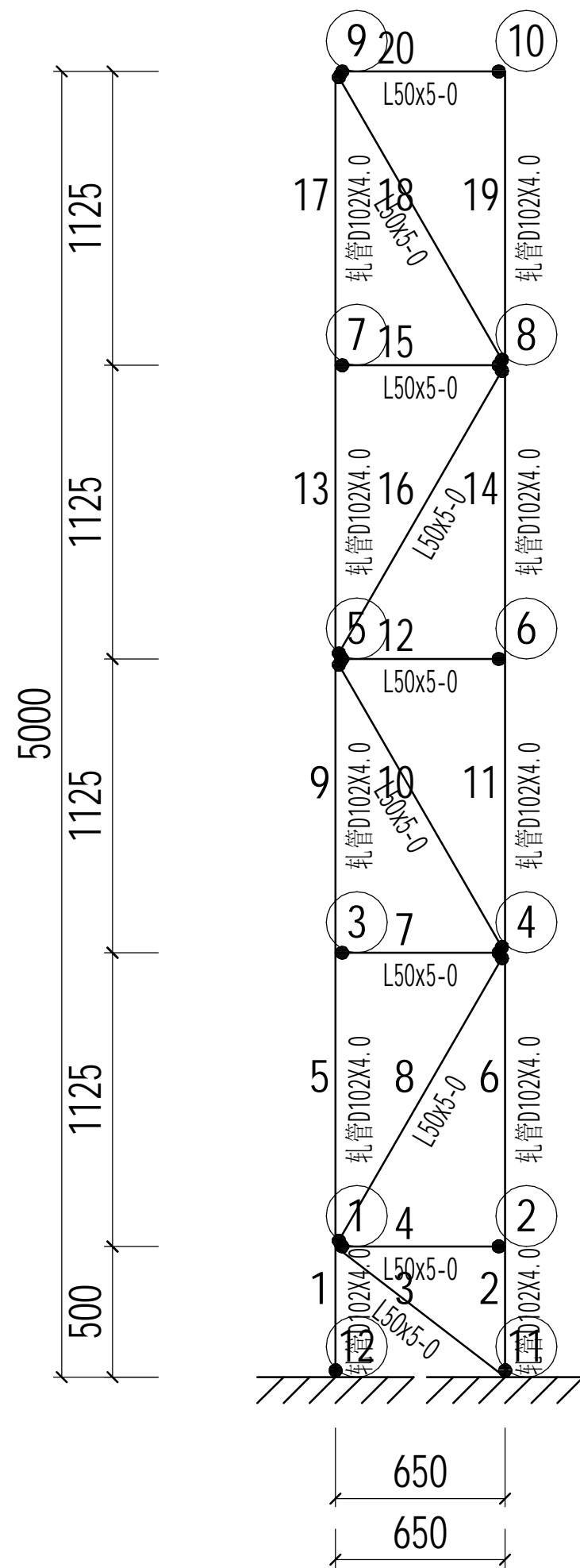
支架立面图 (KLM. T)
